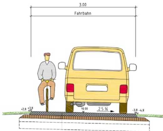
Regelquerschnitt Zufahrtsstraße Aphasie-Zentrum
