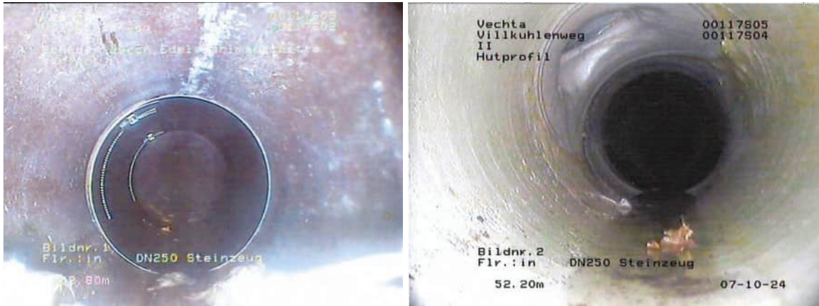
Bild: Sanierung einer Undichtigkeit durch eine Edelstahlmanschette (links), Sanierung eines Stutzens durch einen Langliner und ein Hutprofil
