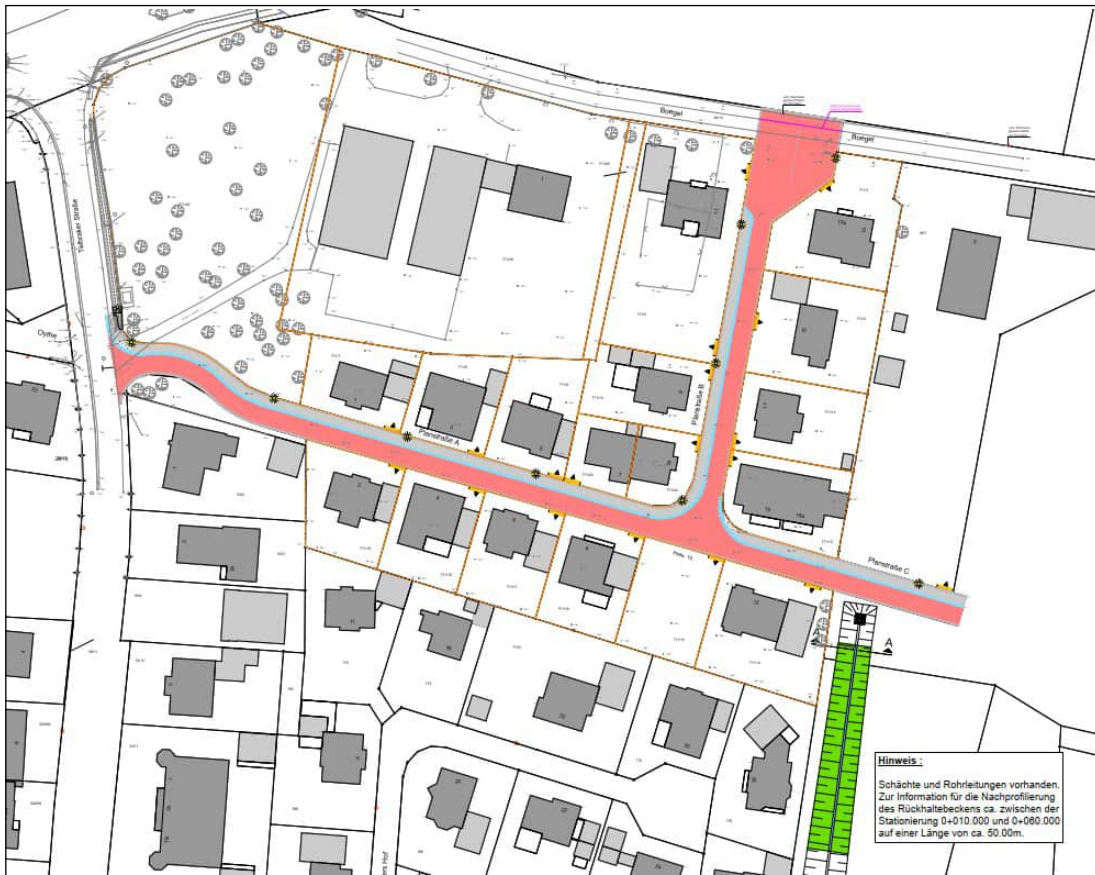
Lageplan
